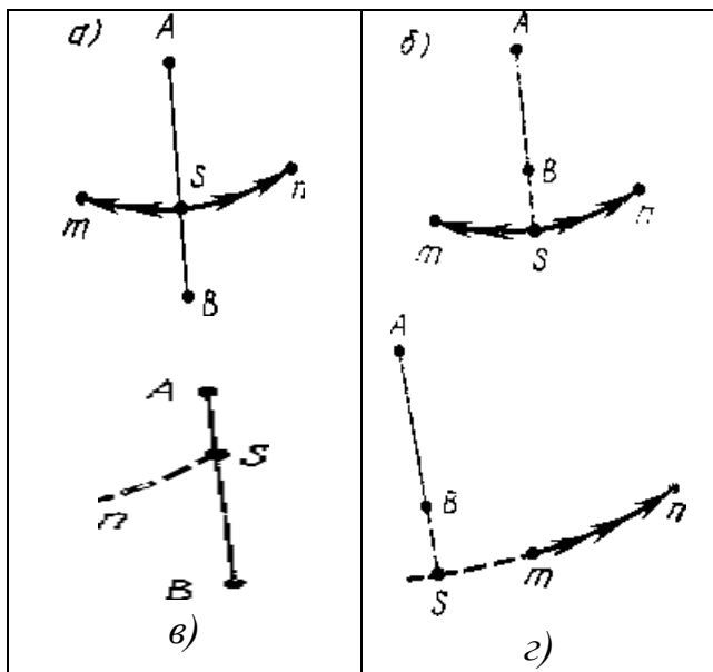
Рис. 49. Возможные случаи взаимного расположения пограничной кривой m\pi и соответствующей ей соединительной прямой AB
