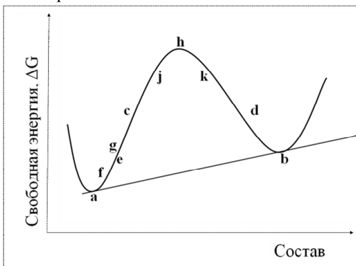
Рис. 63. Схематическая кривая зависимости свободной энергии от состава в системе с расщеплением
