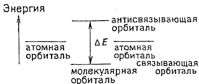
Рис. 4. Молекулярные орбитали в двухатомной молекуле
